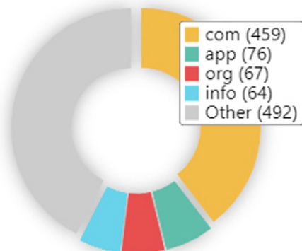
Top TLDs
